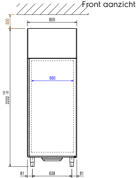
Zij aanzicht
